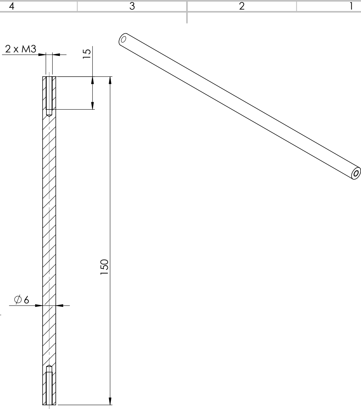
COUPE A-A
