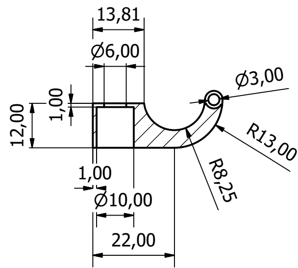
A-A ( 1 : 1 )
