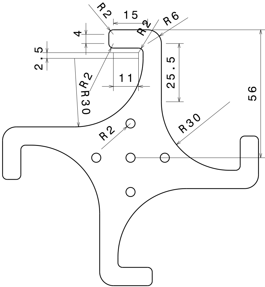
Vue de face Echelle : 1:1
