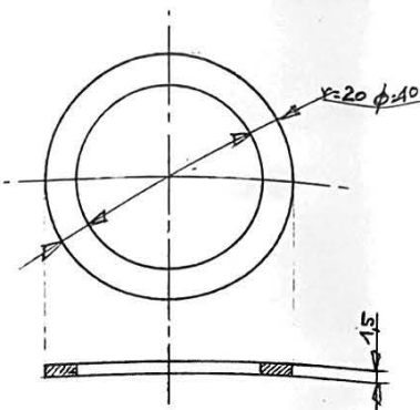
2 Bagues Bronze de frottement
