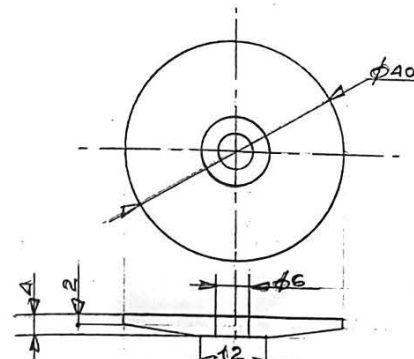
Bague inférieure
