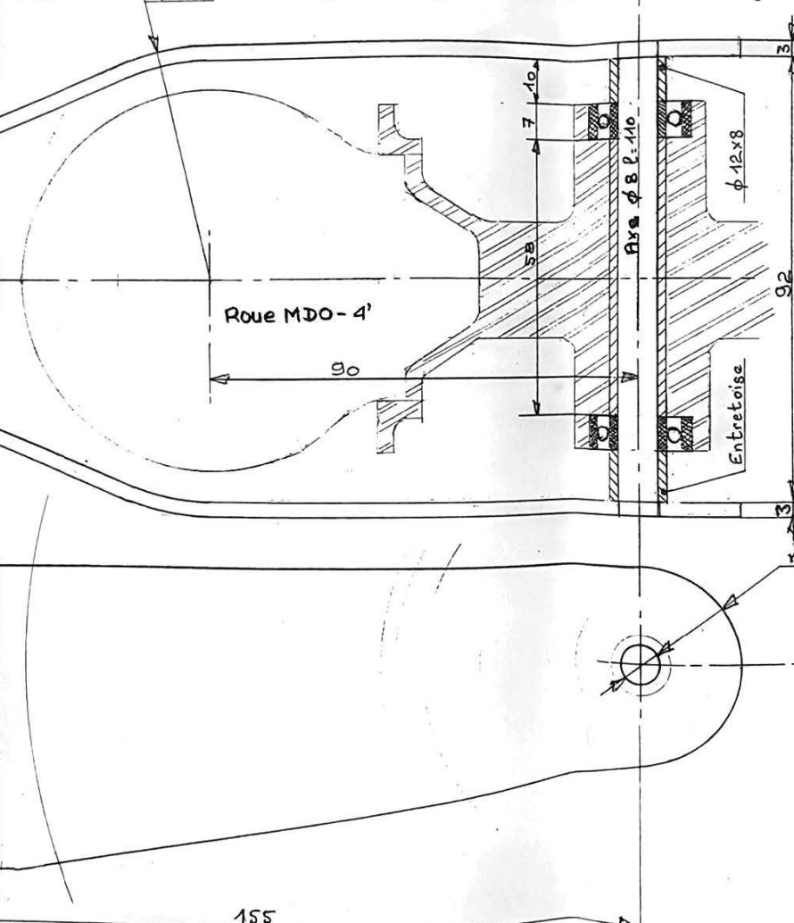
2 Bagues Bronze de frottement
