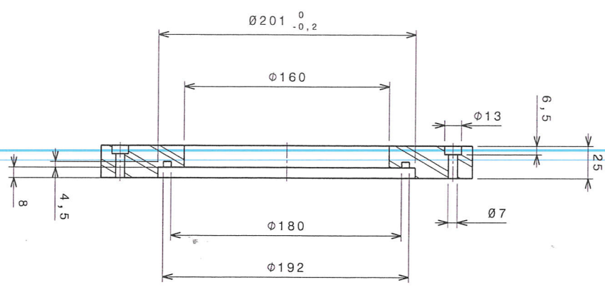
Coupe A-A Echelle : 1:2
