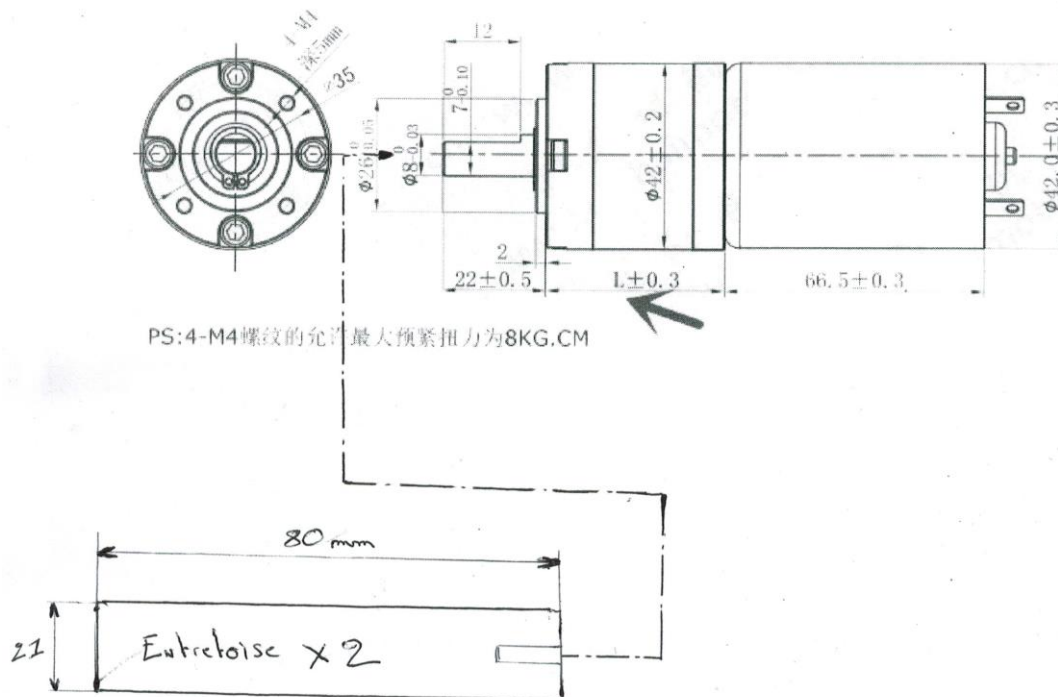
外形图(Outline Drawing)
