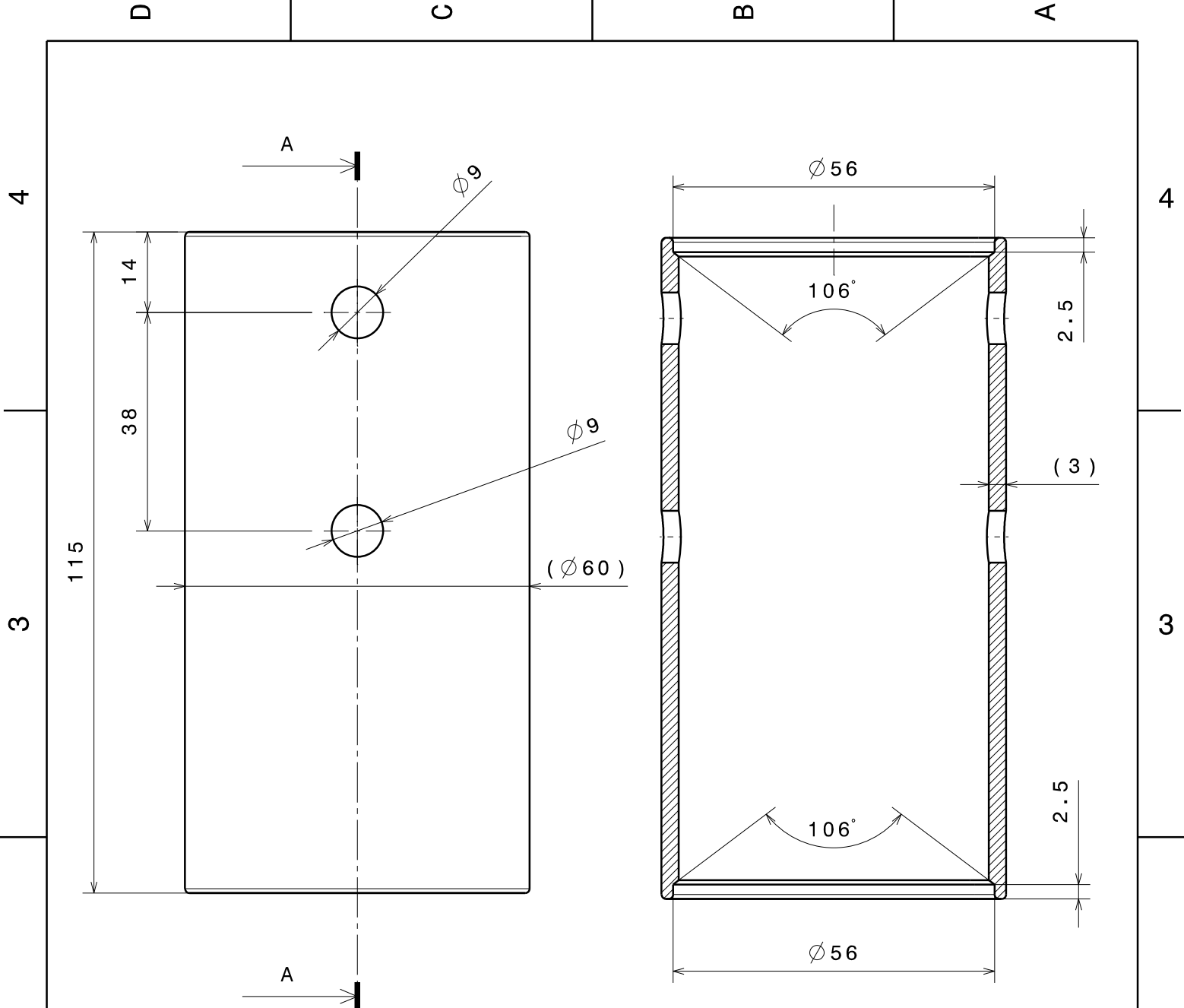
Vue de face Echelle : 1:1
