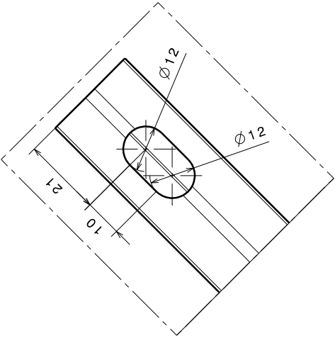
Vue auxiliaire A Echelle : 1:1
