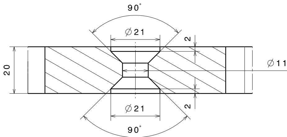
Coupe A-A Echelle : 1:1
