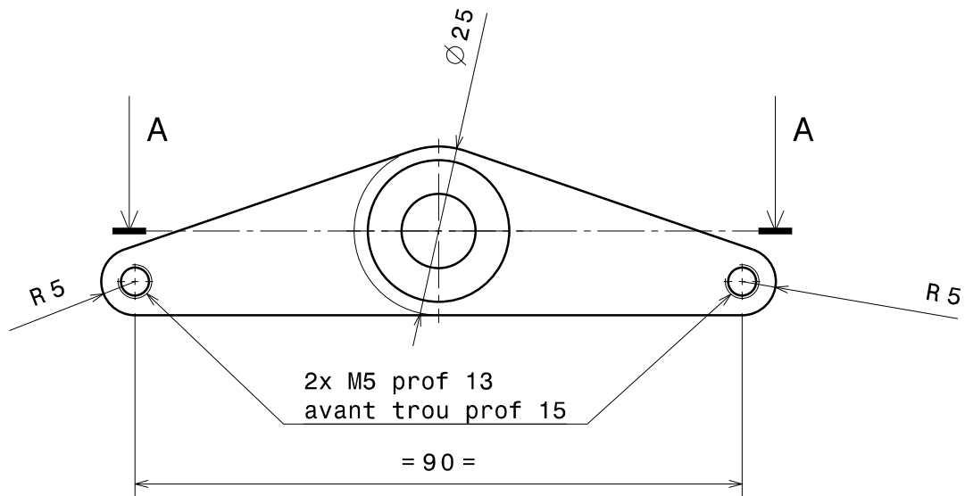
Vue de face Echelle : 1:1
