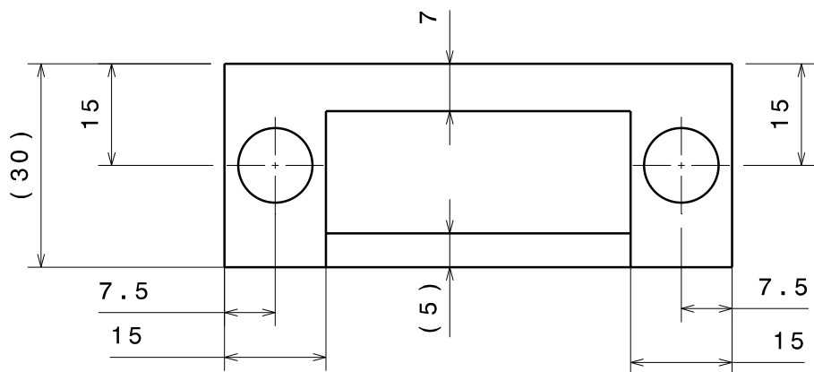
Vue de dessus Echelle : 1:1
