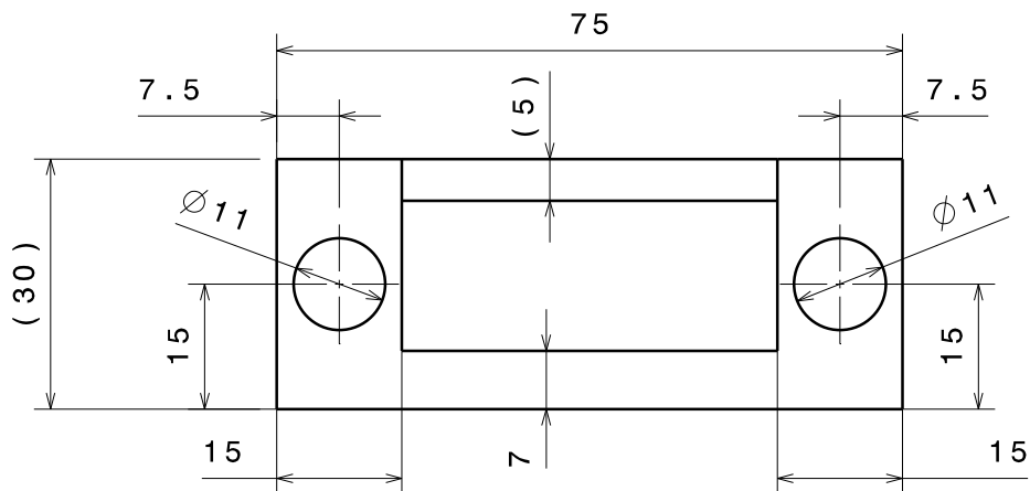
Vue de face Echelle : 1:1
