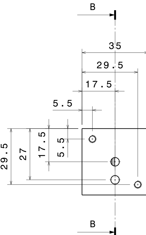
Vue de gauche Echelle : 1:1
