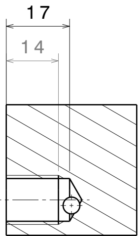
Coupe C-C Echelle : 1:1
