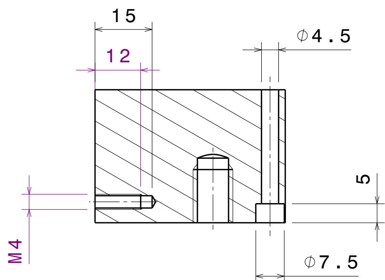
Coupe E-E Echelle : 1:1
