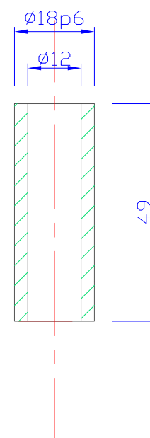
Rep7 - Embouts tuyaux Matériau: INOX Quantité: 2
