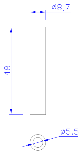
Rep6 - Support vérin Matériau: INOX Quantité: 4
