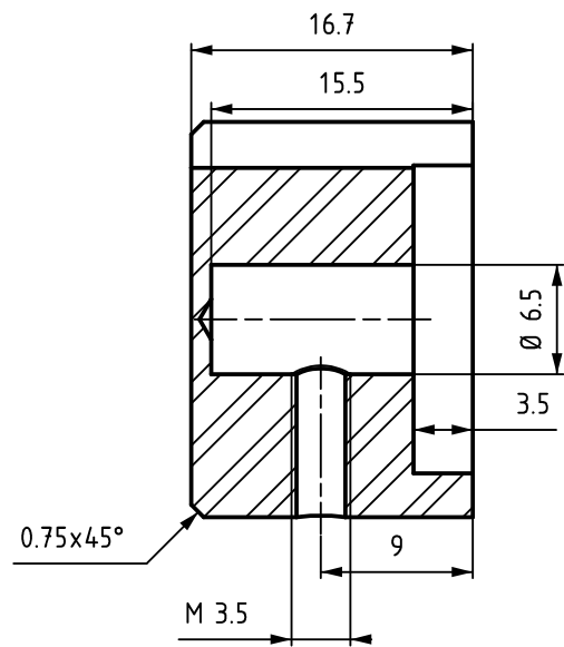
Coupe A-A
