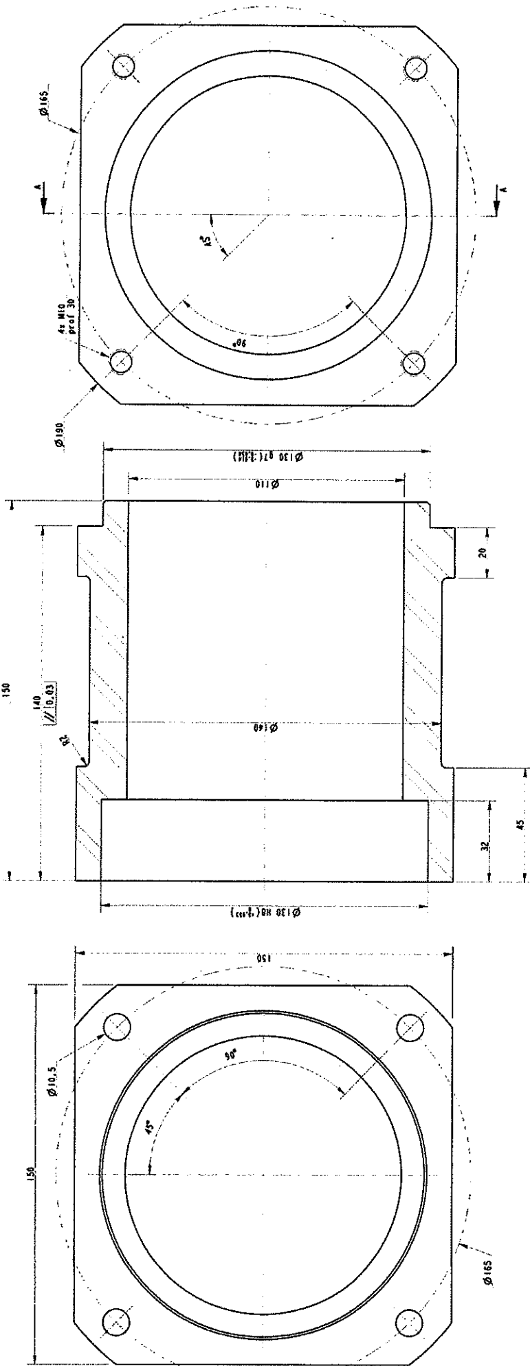
COUPE A-A
