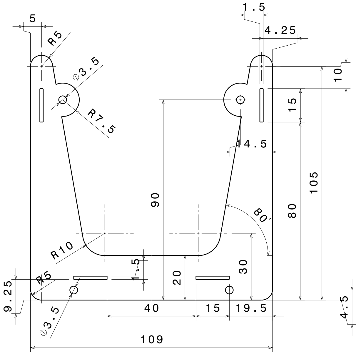
Vue de face Echelle : 1:1
