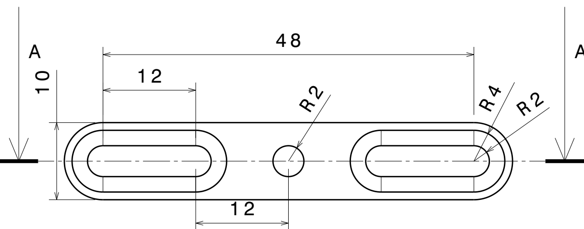
Vue de devant Echelle : 2:1
