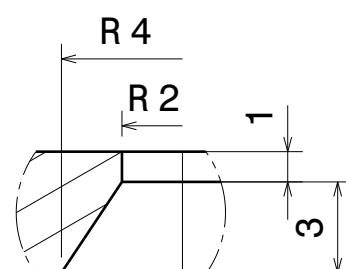
Détail C Echelle : 4:1
