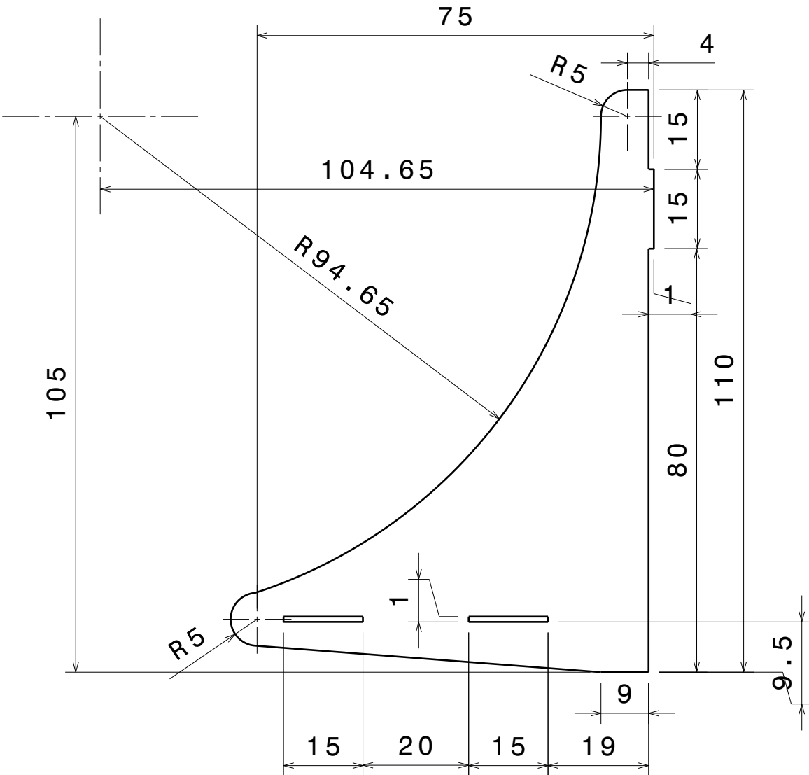
Vue de face Echelle : 1:1
