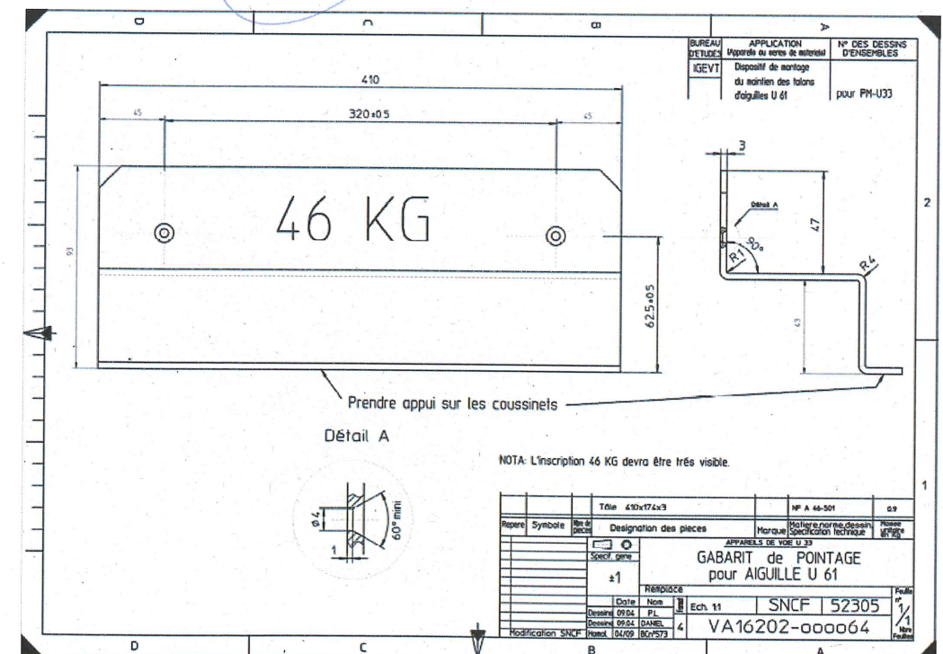
Dessin VA 16202-000064 Gabarit de pointage pour une aiguille 46 kg
