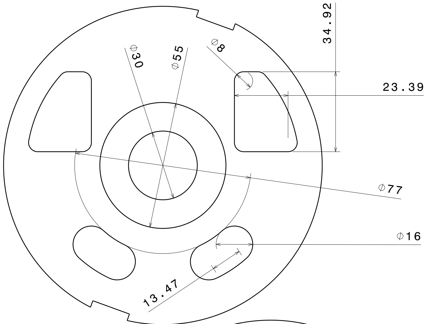
Vue de face Echelle : 1:1
