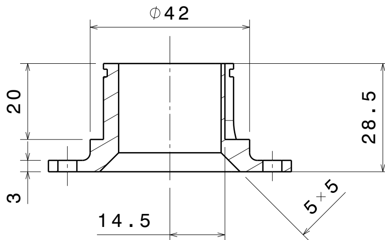
Coupe A-A Echelle : 1:1
