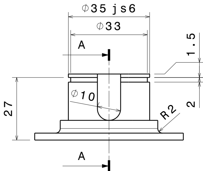
Vue de face Echelle : 1:1
