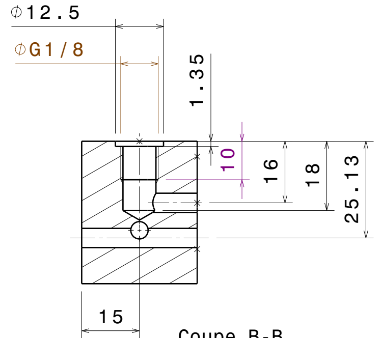
Coupe B-B Echelle : 1:1
