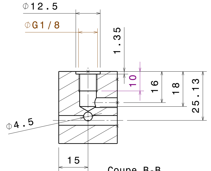
Coupe B-B Echelle : 1:1
