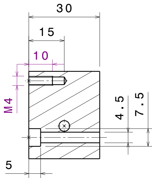
Coupe C-C Echelle : 1:1
