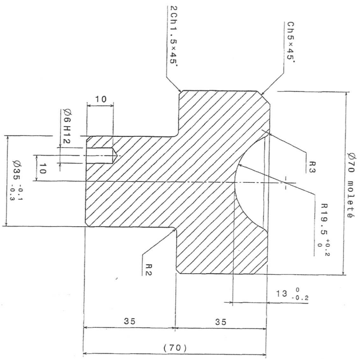
Coupe A-A
