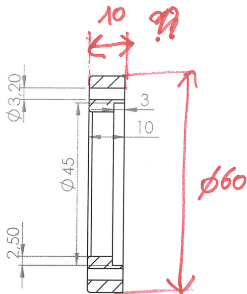
COUPE A-A
