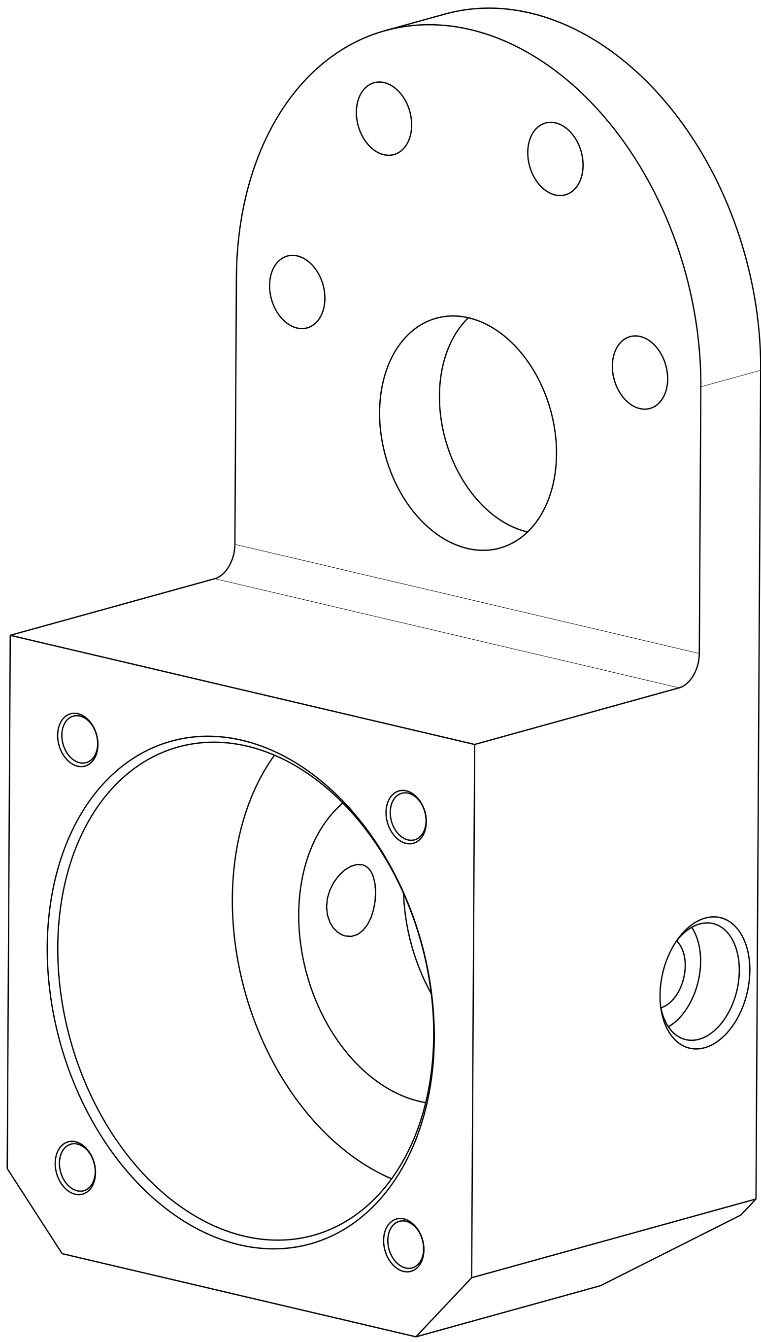
Vue isométrique Echelle : 4:1
